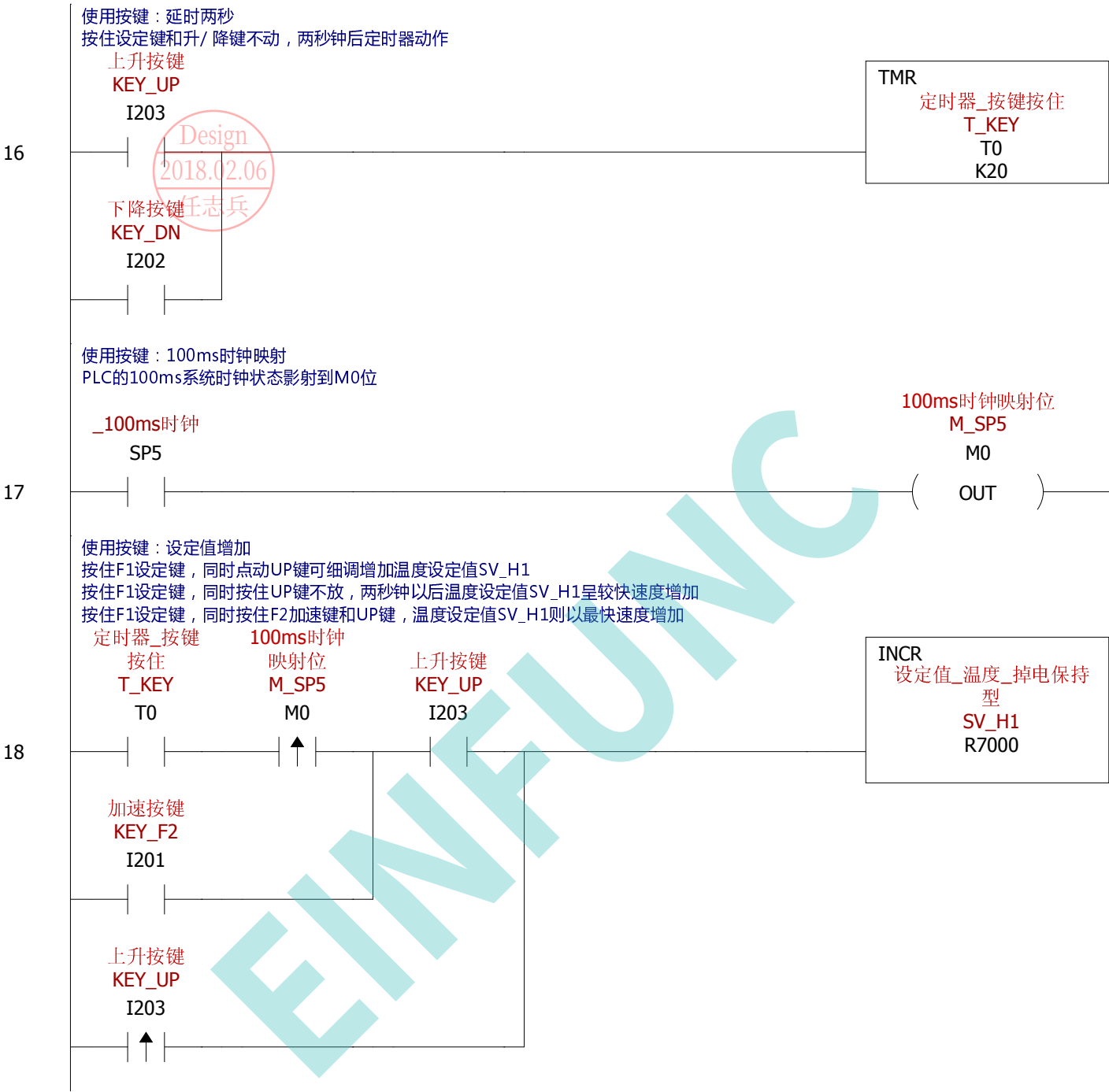
梯形图视图
