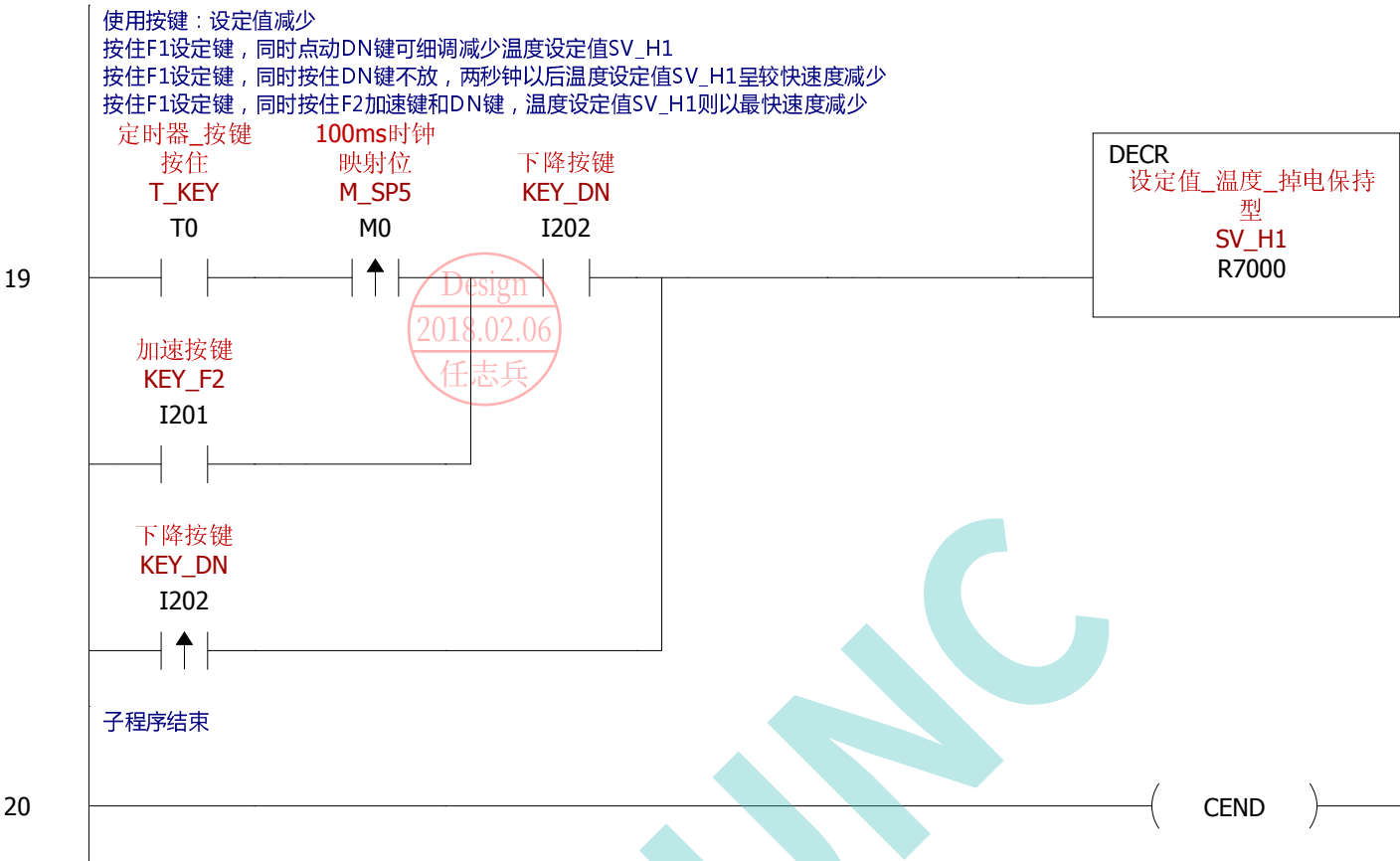
梯形图视图
